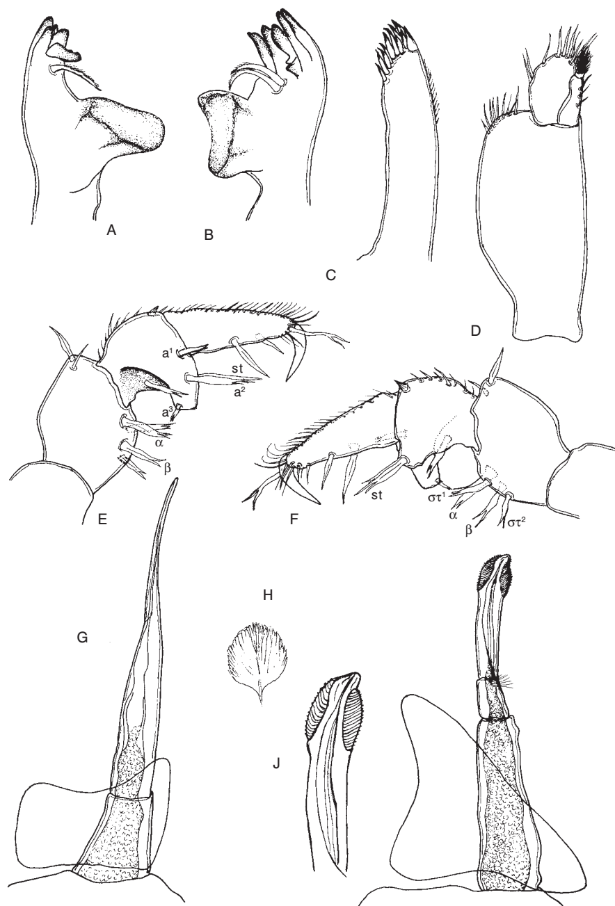
Fig. 2. Alistratia beroni n. gen. n. sp., holotype \sigma : A – mandibule gauche; B – mandibule droite; C – maxillule, endit externe; D – maxillipède; E – péréiopode VII, face interne; F – péréiopode VII, face externe; G – pléopode II; H – soie écaille. I – pléopode I; J – pléopode I à un grossissement plus fort
